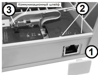
Рис. Ж.1 Порядок установки адаптера
