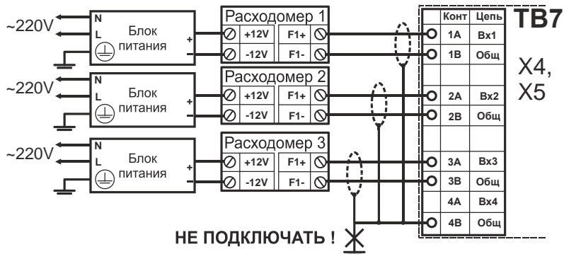
Рис. 4.2 Пример подключения импульсных линий связи
